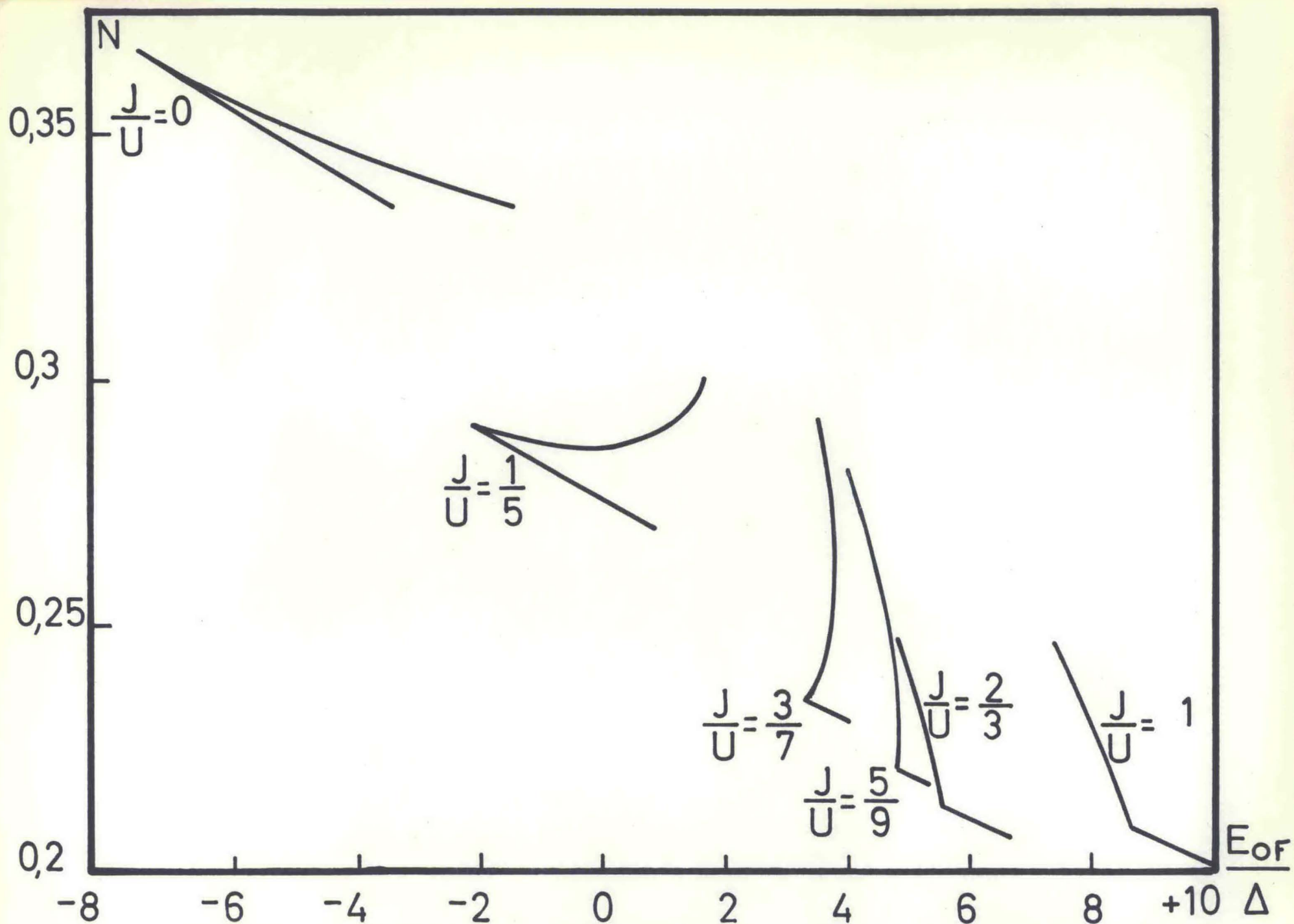
Fig-20: Nombre total d'électrons au voisinage de la condition de découplage d'orbite pour différentes valeurs de \frac{J}{U} et à une température donnée kT = 8\Delta
